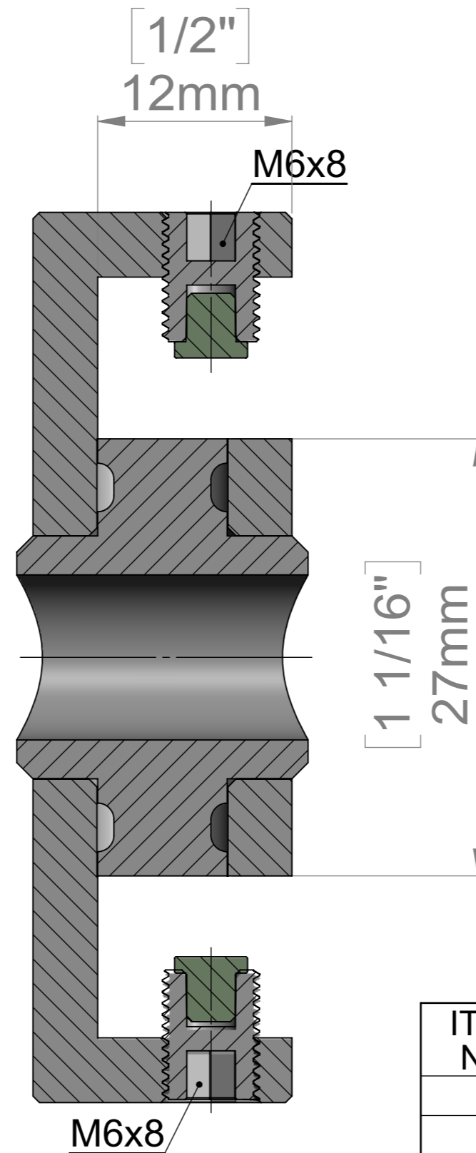
SECTION A-A SCALE 3 : 1
