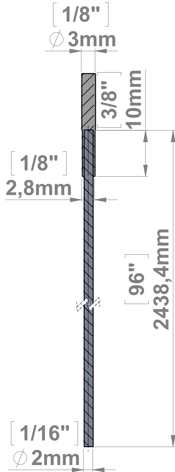
SECTION A-A SCALE 2:1
