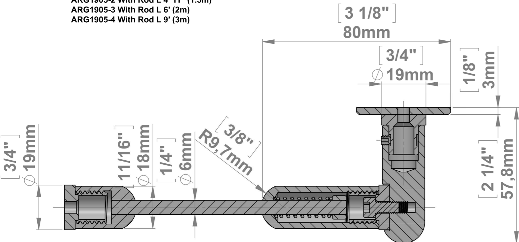
SECTION A-A SCALE 1 : 1
